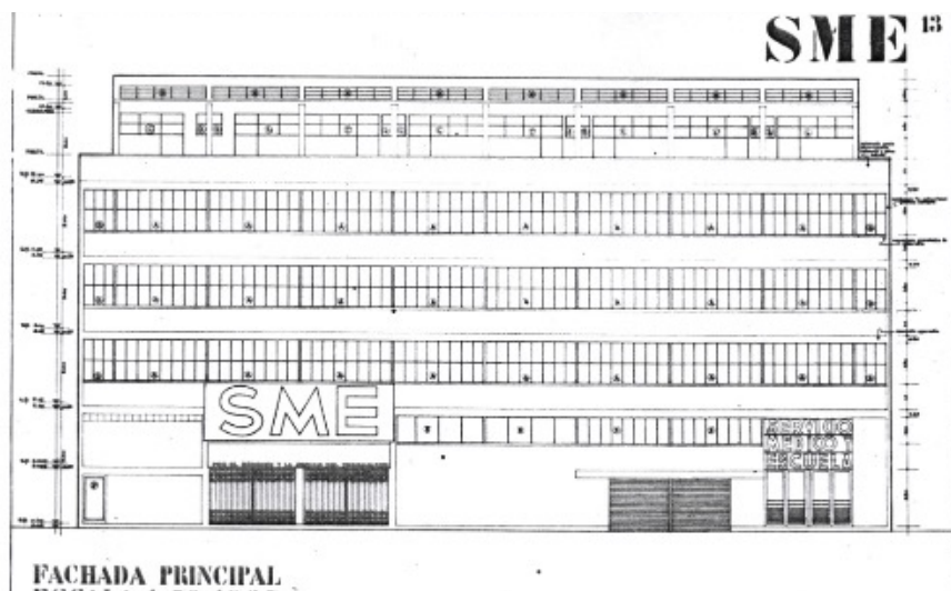
Plano de la fachada de la nueva sede del SME en Artes 45, del Arq. Enrique Yáñez (1937)
